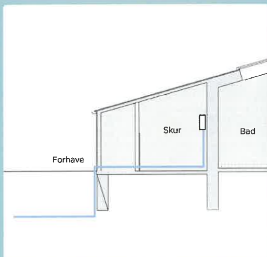
Hovedvandleddningen kommer op ad jorden foran skuret og bliver så ført ind gennem skuret og hen til vand- og varmeanlægget på væggen.
