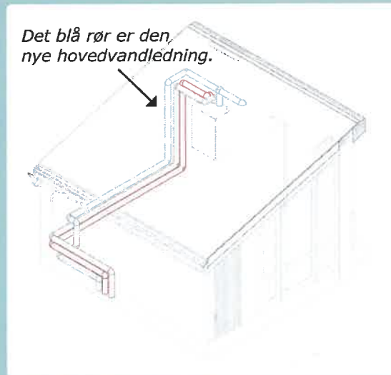
Det blå rør er den nye hovedvandleddning. Eksempel på føringen af nye vandrør i skuret.
